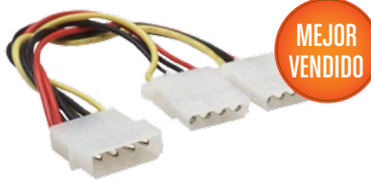
301503. Cable de alimentación interna en "Y" Molex 1 a 2
